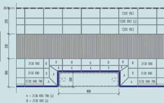
Узел 2
