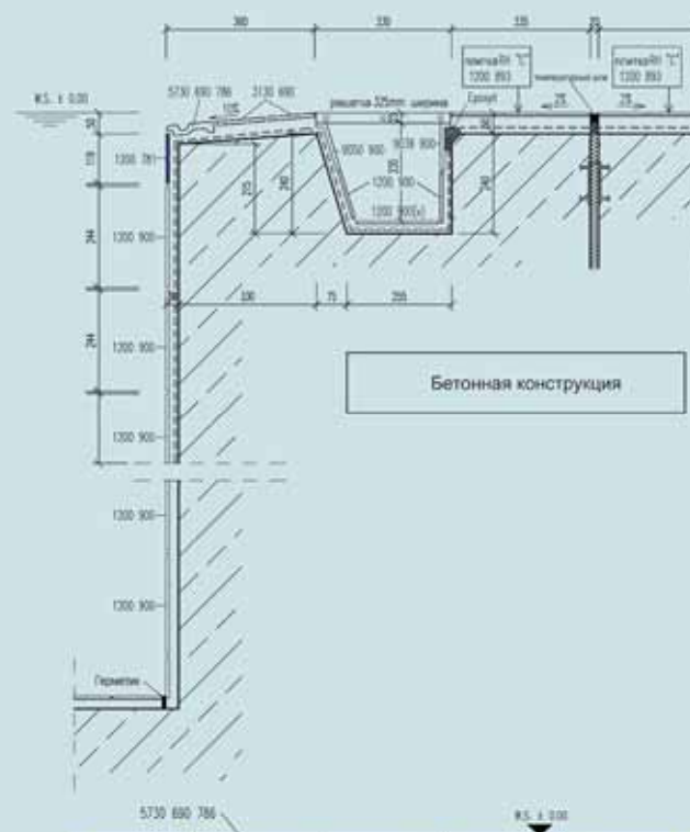
Узел 1
